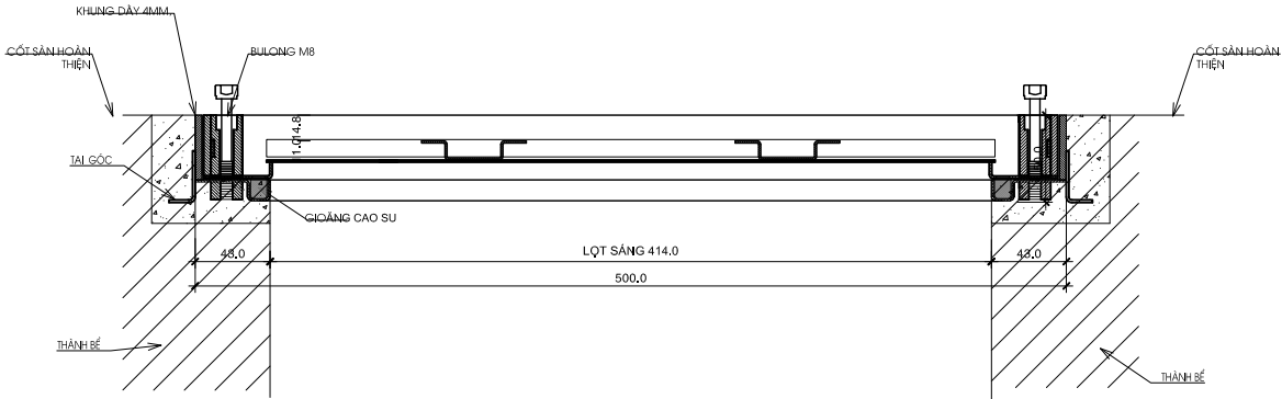
MẶT CẮT
