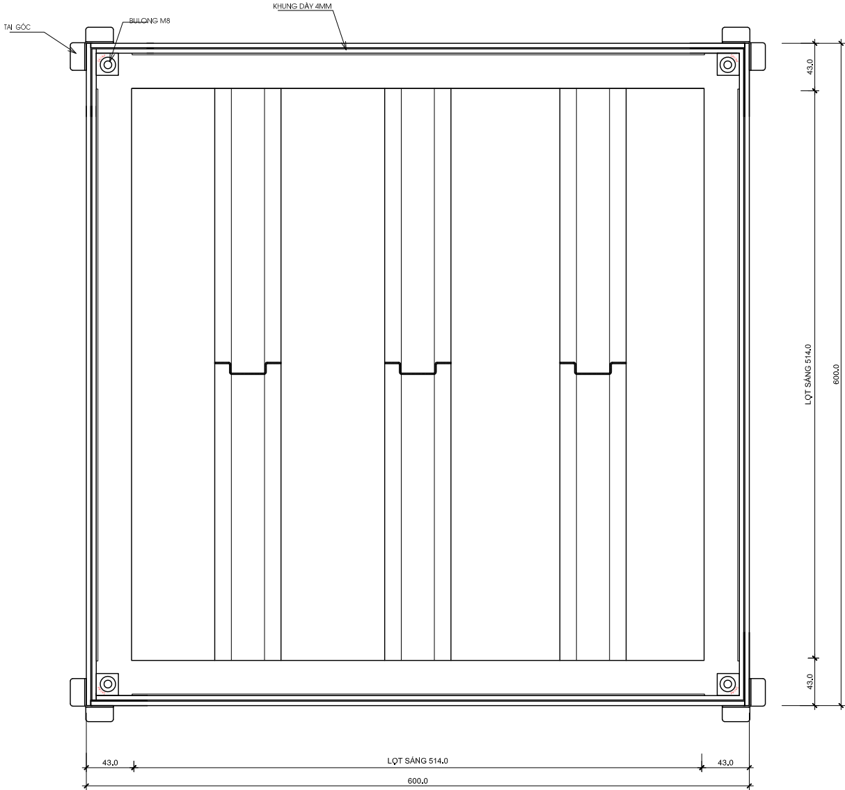
MẶT BẰNG
