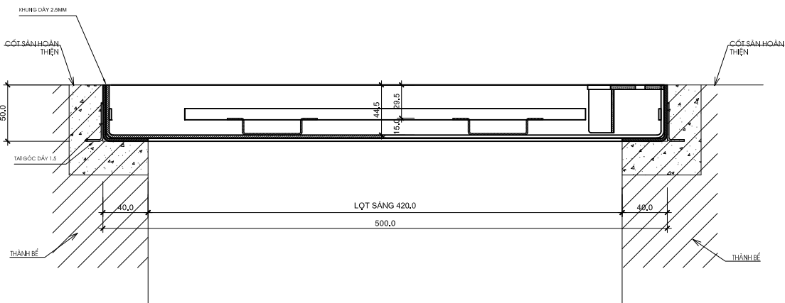
MẶT CẮT
